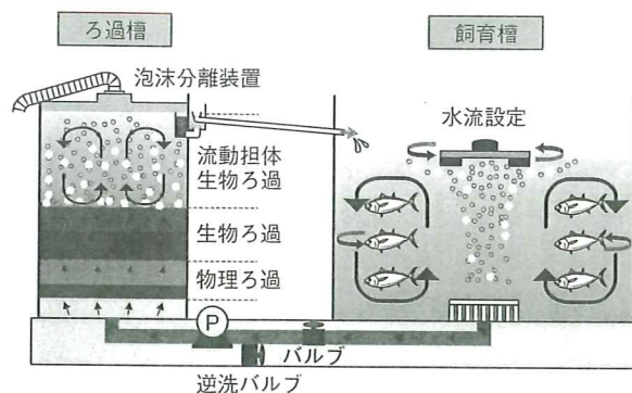
新たに泡沫分離装置を標準装備したろ過システムのフロー図
